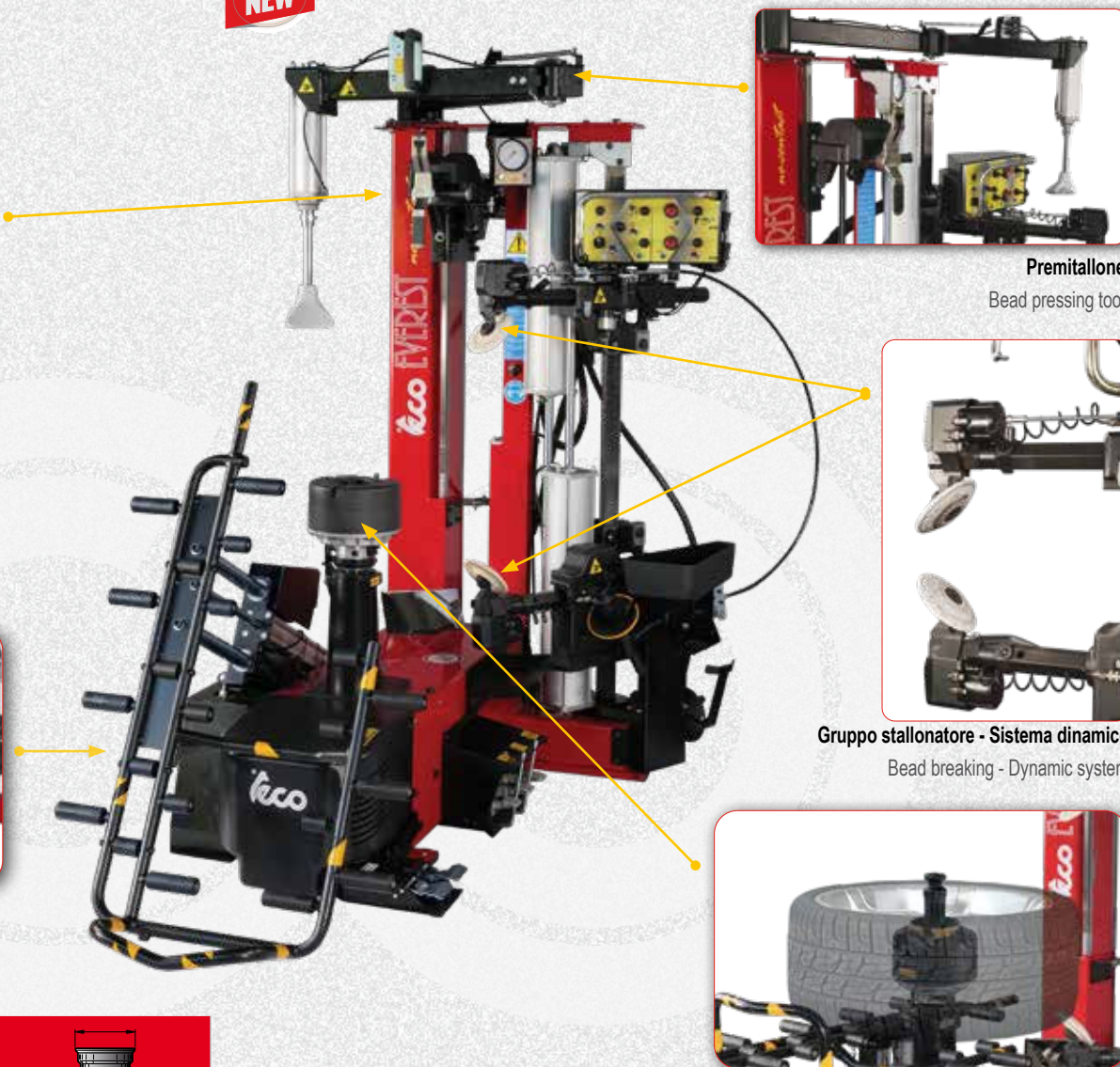
Autocentrante con bloccaggio automatico Automatic axial mounting shaft-pneumatic
